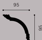
WT11 WALLSTYL®
